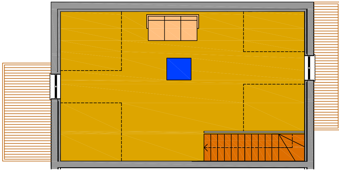
VIVIENDA TIPO 6 - PLANTA BAJO CUBIERTA Sup. Útil 27.50 m 2
